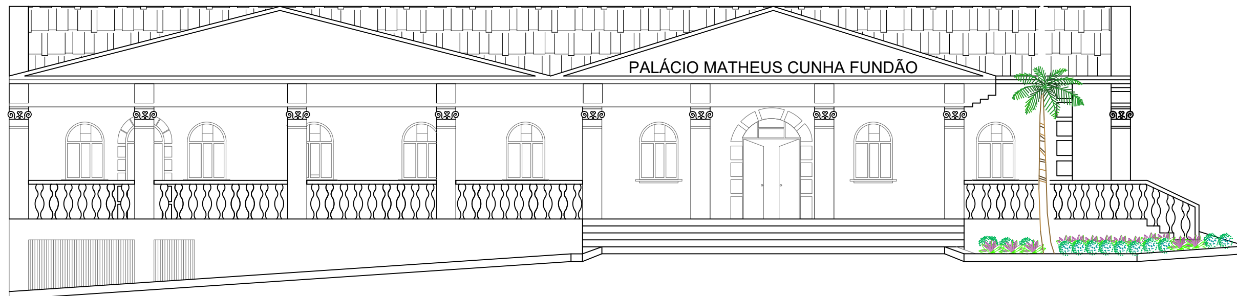
FACHADA FRONTAL sem escala
