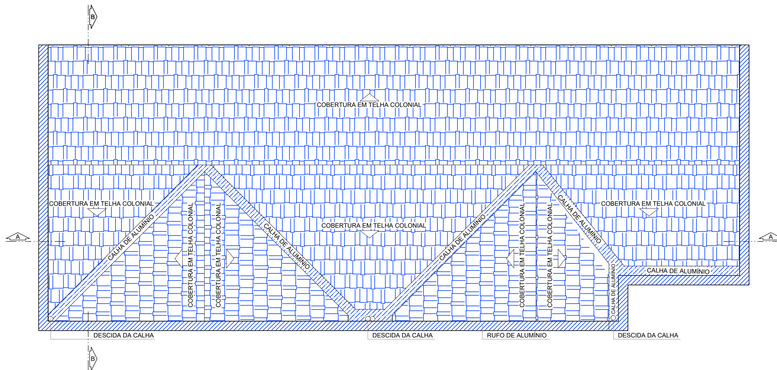
PLANTA DE REFORMA DA COBERTURA esc 1:100
