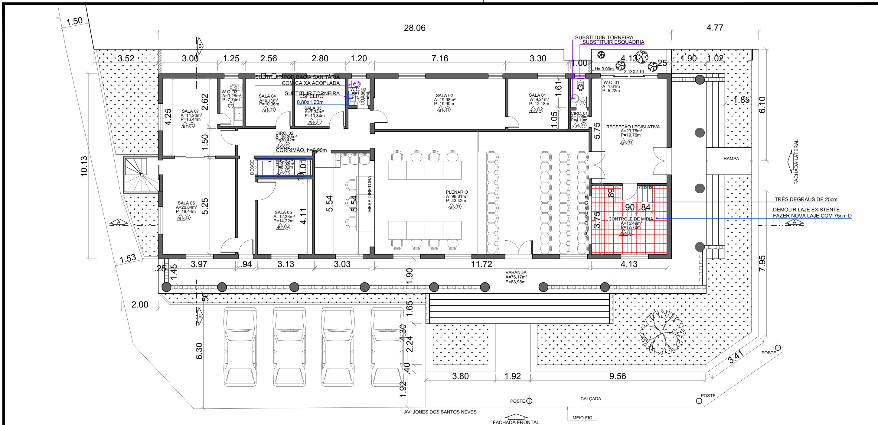
PLANTA BAIXA DE REFORMA PAVIMENTO TÉRREO esc 1:125
