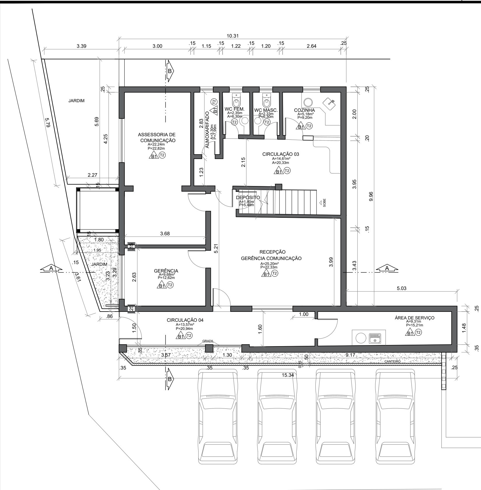
AV. JONES DOS SANTOS NEVES PLANTA BAIXA DE REFORMA PAVIMENTO INFERIOR esc 1:100
