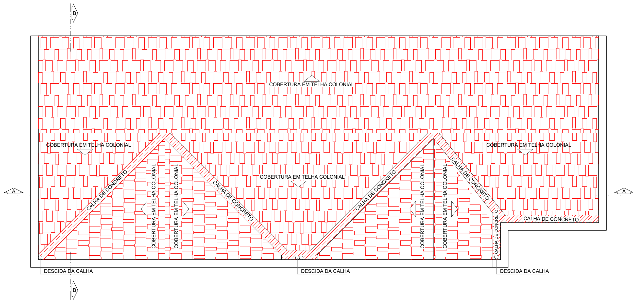
PLANTA DE COBERTURA ATUAL esc 1:100
